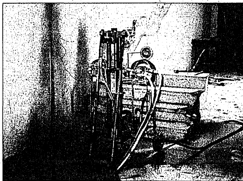
Entfernung eines Treppenfundaments mit einer speziellen Seilsäge.
