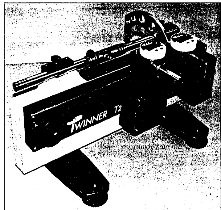
TWINNER ist ein Messgerät als multifunktionales Messzentrum auf dem (fast) alles was auf einer Drehmaschine entsteht, vermessen und dokumentiert werden kann.
