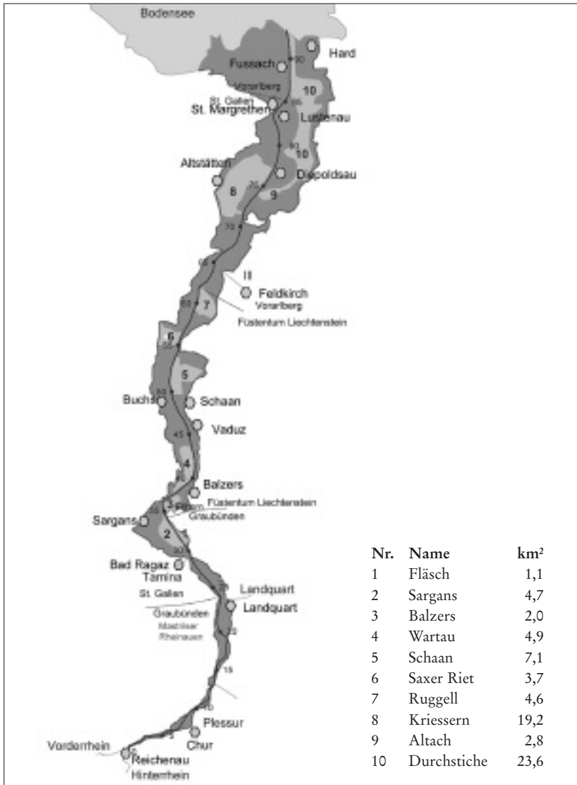
Abbildung 4: Das Entwicklungskonzept stellt für den Alpenrhein 10 Notentlastungsräume zur Diskussion (dunkelgraue Flächen). Sie sind die «Ultima Ratio», das letzte Mittel, wenn es im ultimativen Katastrophenfall darum geht, den unvermeidlichen Schaden so gering wie möglich zu halten. (Grafik: Zarn/ARGE Rheinblick)
