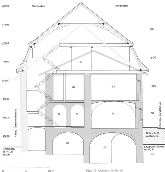
Plan 17: Querschnitt durch den Gasthof von 1776, 1:100; in dunklem Grauton der Kernbau des 14. Jahrhunderts, in hellem Grauton die Erweiterung von 1666
