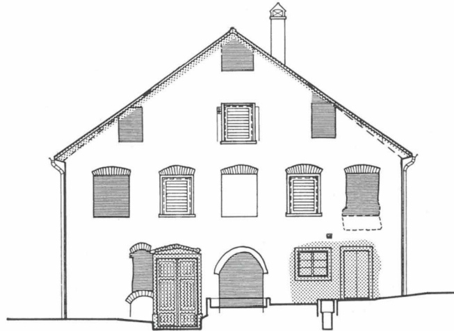
Abb. 36: NO-Fassade
