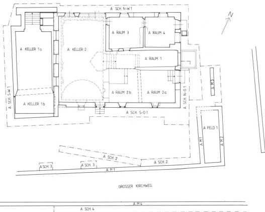
Abb. 4: Schnitte, Mauern, Kellergeschoss
