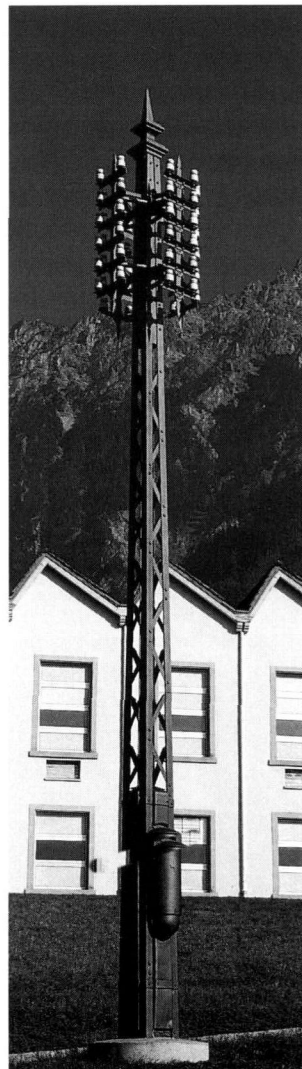
Abb. 5: Historischer Telefon-Freileitungsmast aus dem «Unteren Mühleholz» in Vaduz. Reinigung und Konservierung im Januar 1995.
