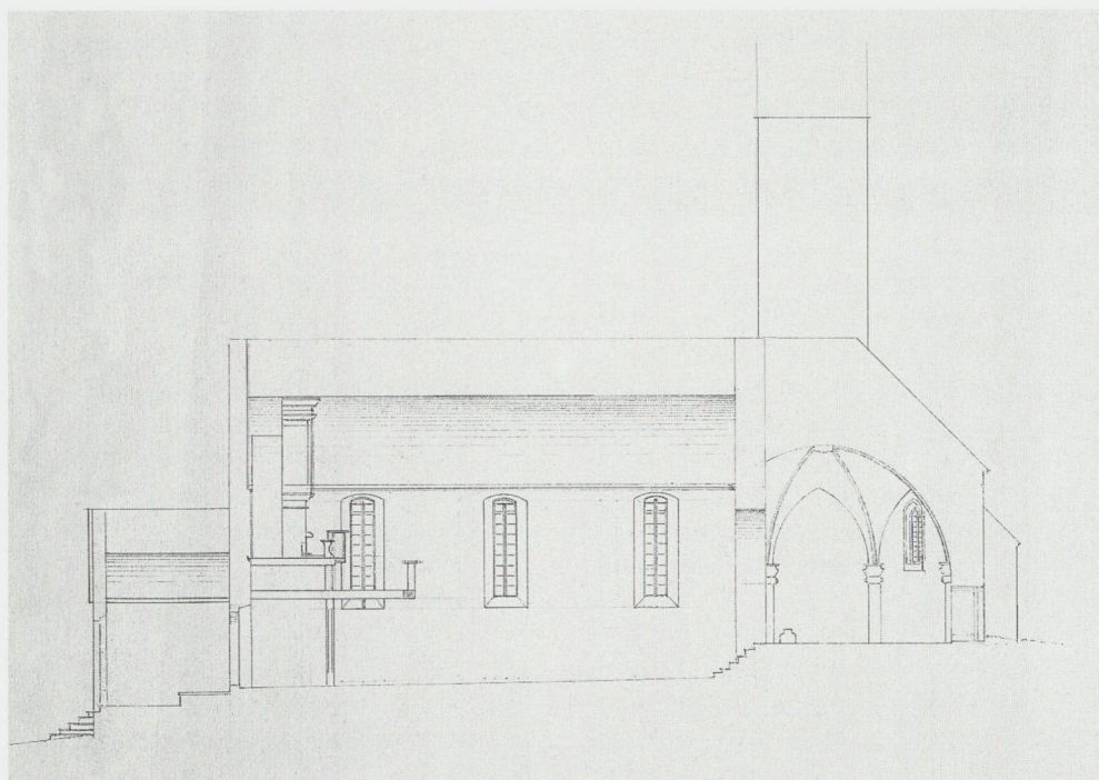
Abb. 3: Längsschnitt durch die Florinskapelle. Blick von Süden. Zweistöckige Orgelempore und Tonnengewölbe im Kirchenschiff, Rippengewölbe im Chor. Bleistiftzeichnung von Landestechniker Peter Rheinberger aus der Zeit um 1870/72.
