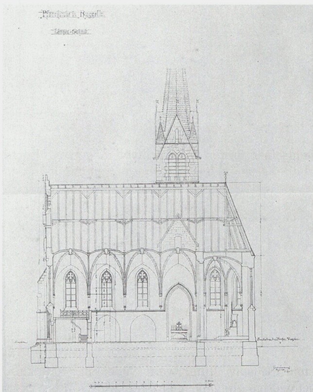
Querschnitt mit Blick nach Westen, Originalplan von 1895
