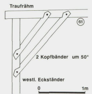
Abb. 18: Abbund der Laube, Südwestansicht, 1:50
