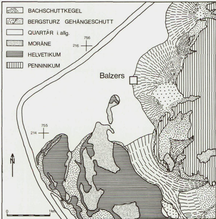
Abb. 13: Geologische Kartenskizze der Umgebung von Balzers; umgezeichnet und vereinfacht nach ALLEMANN (1985).
