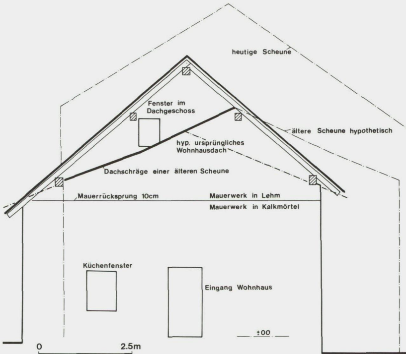
Abb. 25: Wohnhaus-Ostfassade, 1 : 100, mit Eintrag der heutigen und einer älteren Scheune.
