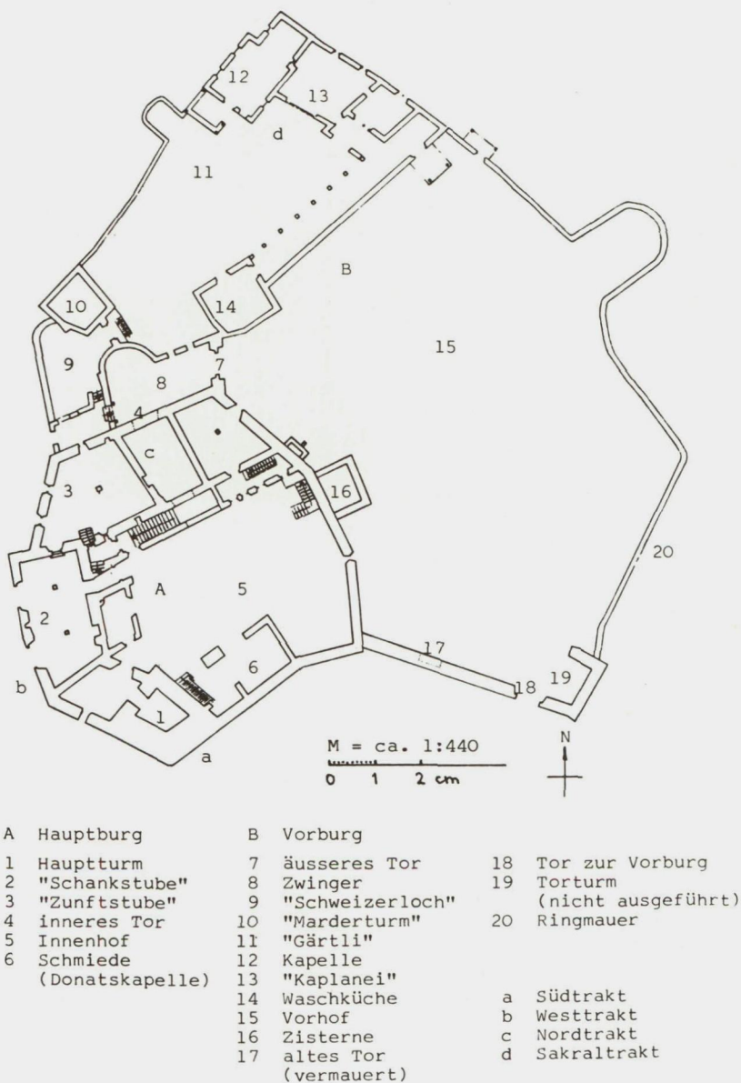
Abb. 50 Burg Gutenberg in Balzers. Grundriss, Neuvermessung 1982.
