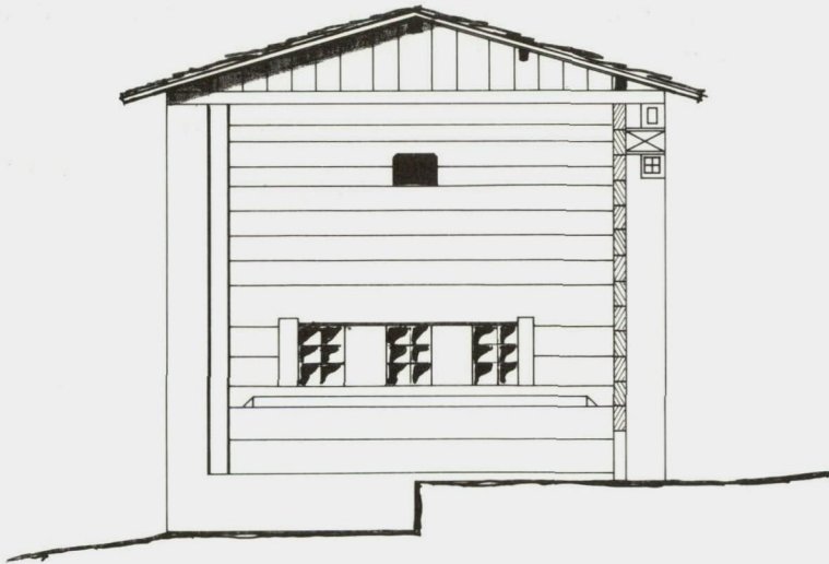
Südfassade Rekonstruktionsversuch aufgrund des vorhandenen Baubestandes.
