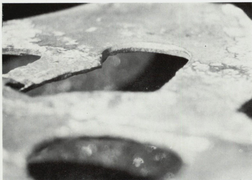
Abb. 5 Typischer Stanzrand mit senkrecht verlaufenden Stanzriefen.
