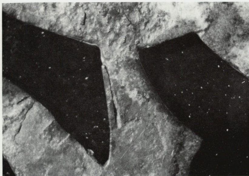
Abb. 6 Hier ist eine vom Stanzrand weg verlaufende Kerbe ersichtlich; diese dürfte bei der Herstellung der Scheibe durch ein leichtes Abrutschen des Loch-eisens oder beim Entfernen des Stanzgrates entstanden sein.
