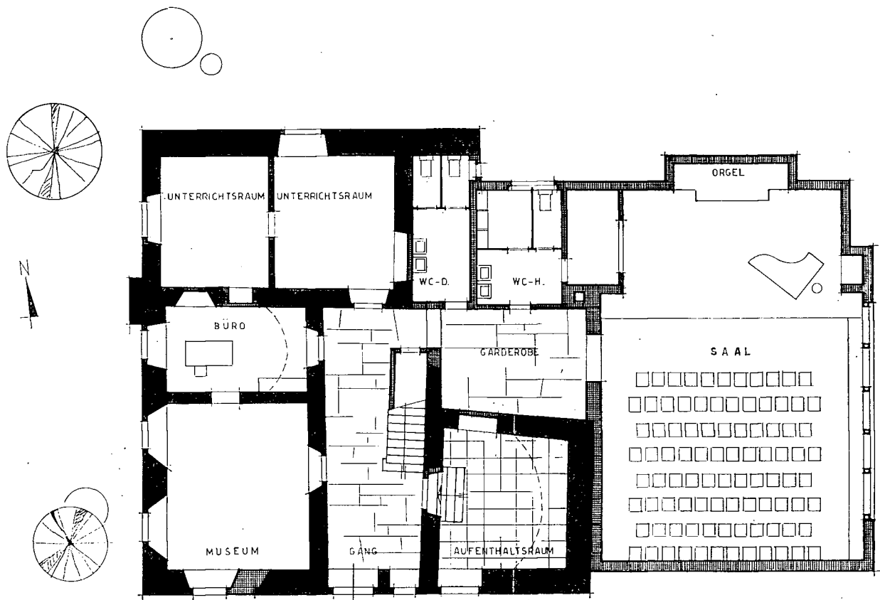
ERDGESCHOSS - NACH DEM UMBAU 1968
