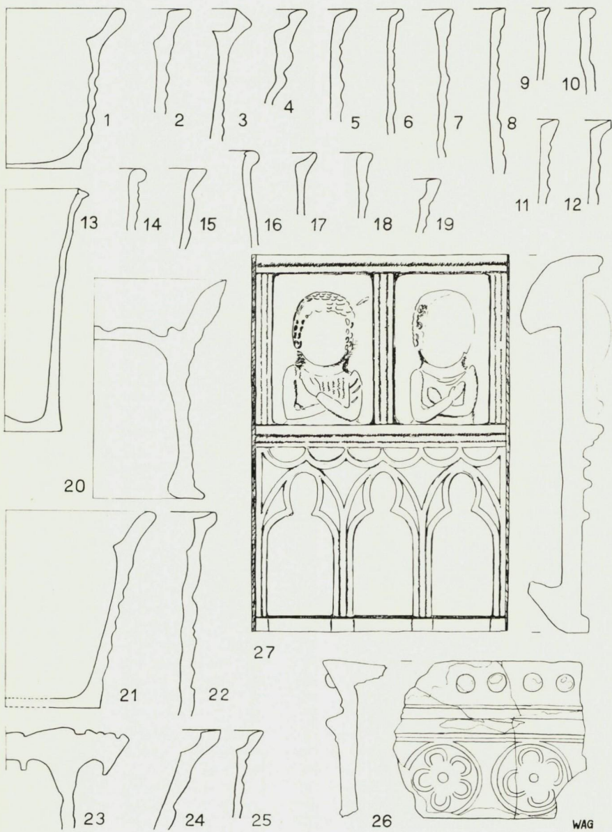
Abb. 32 Profile und Zeichnungen der Ofenkacheln
