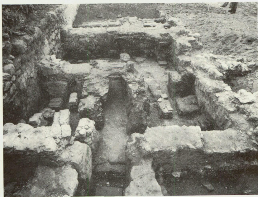
Abb. 7. Das ausgeräumte Kastellbad (Hypokaustum) (Photo Walter Wachter, Schaan)
