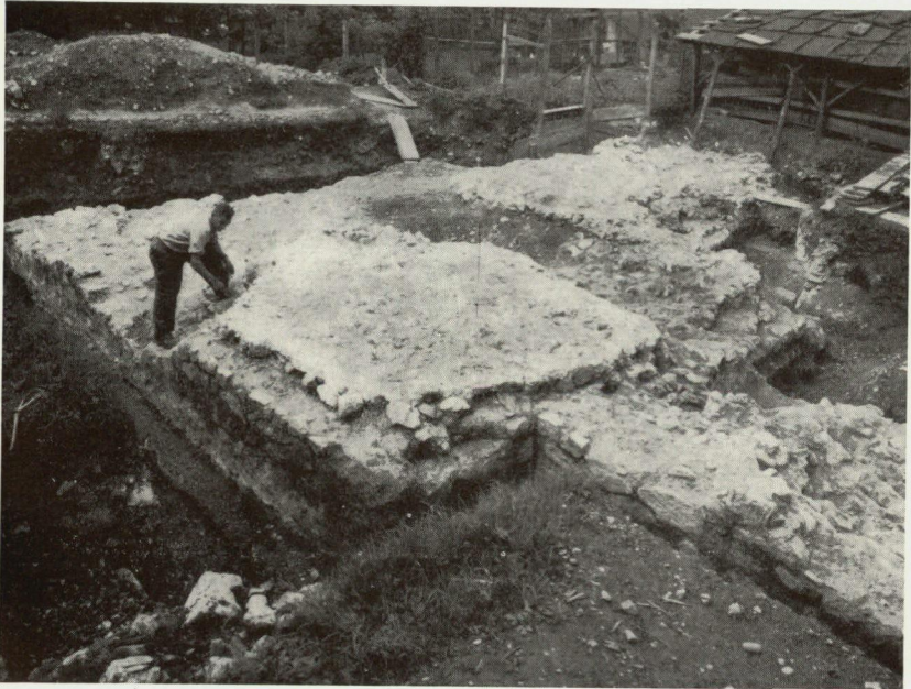
Abb. 5. Der SO-Turm geg. SW, unten rechts die Ostmauer (Photo Walter Wächter, Schaan)
