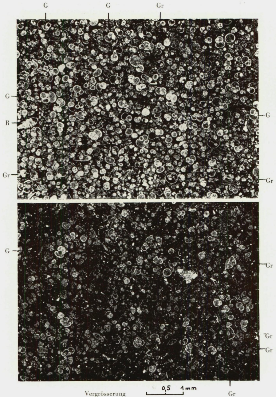
Fig. 1. (oben) Globigerinen-Mergelkalk. Aus den verschleppten Spänen der Falknis-Decke an der Basis der oberostalpinen Heubühl-Scholle. Ca. 1600 m SE Bargella. (G) Globigerina sp. («bulloides-Typ» nach C. A. Wichler) (Gr) Globorotalia sp., (Gr) Reussella .
