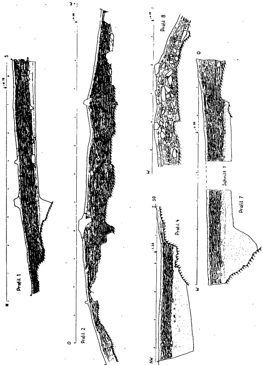
Abb. 3. „Schmeller“, Profile. Legende: Schwarz = jüngere Schicht; stark punktiert = ältere Schicht; leicht punktiert = Löss.
