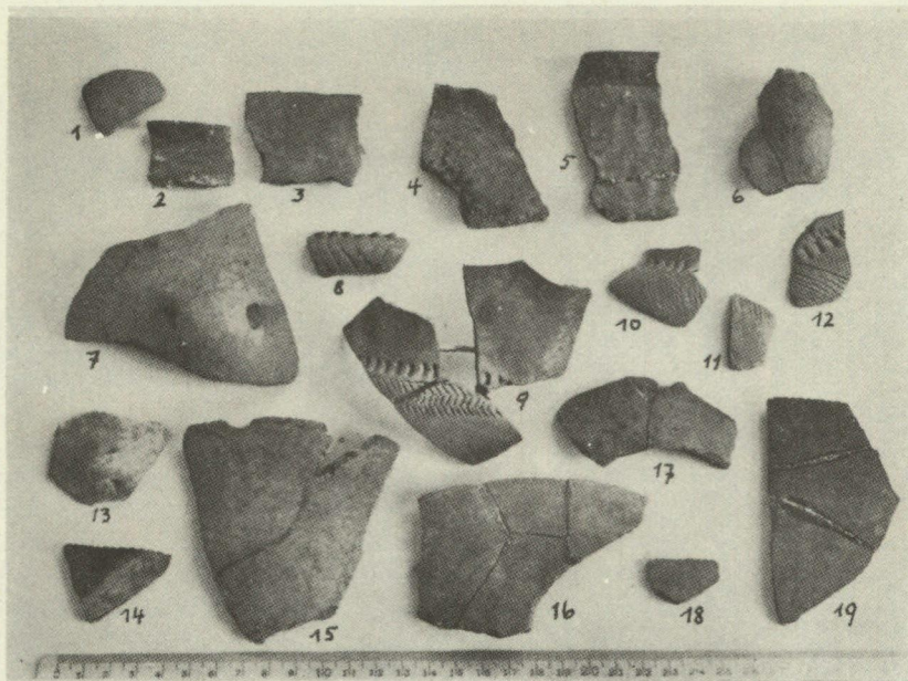
Abb. 9. Rössener Keramik.
