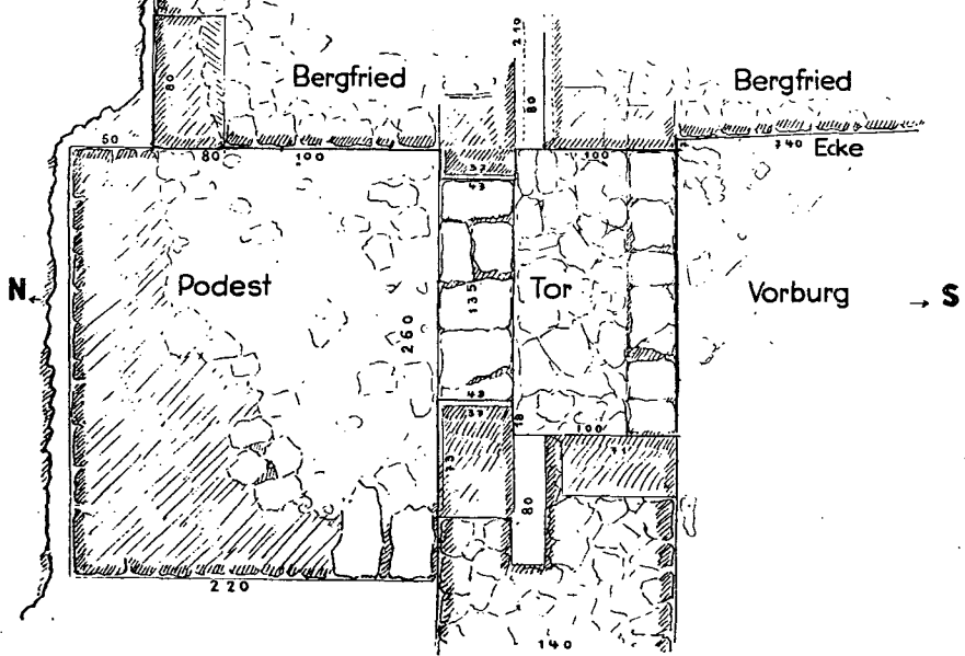
Das Tor zur Vorburg Zeichnung und Grundriß
